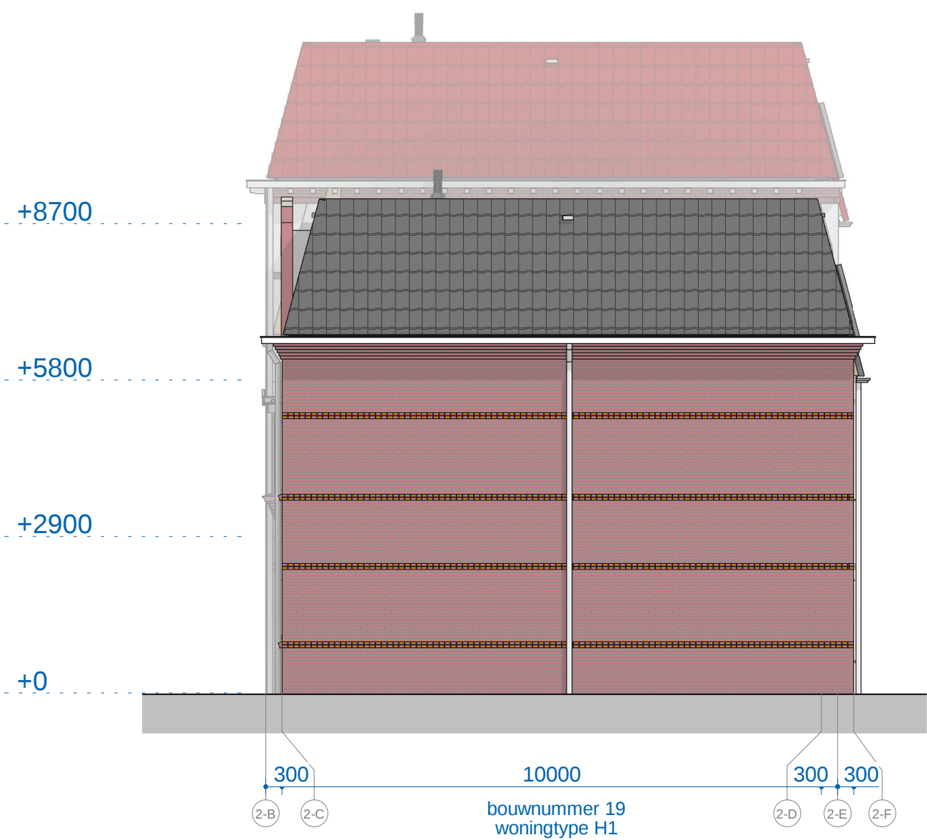
B2_rechtergevel
